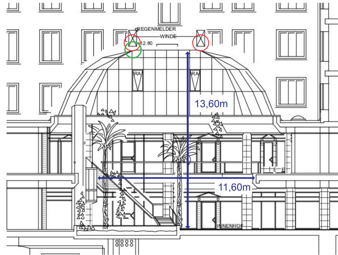
Längsschnitt
